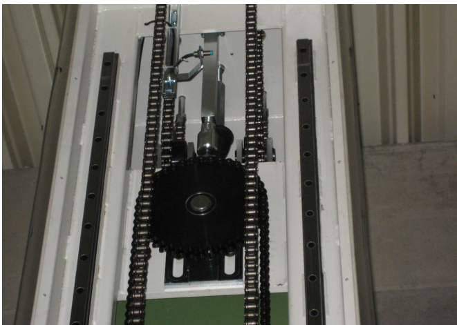
Automatische Kettenspannung
